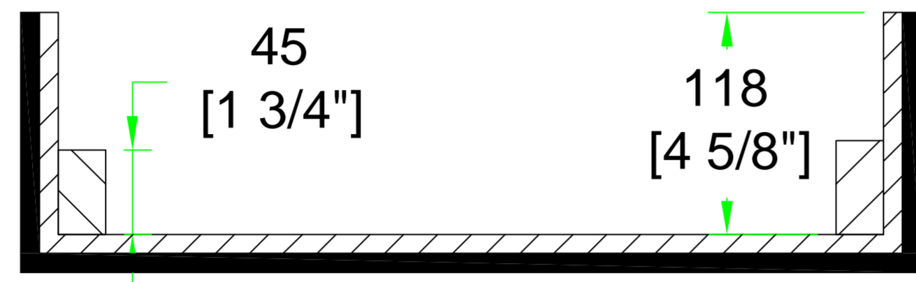
A-A VIEW
