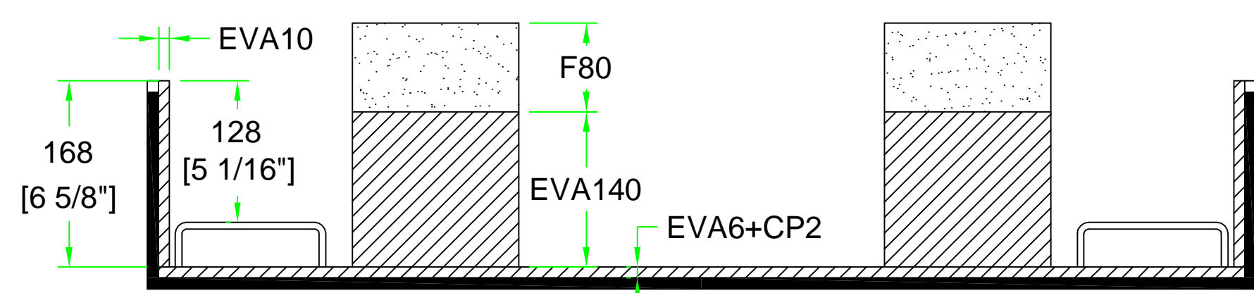
A-A VIEW
