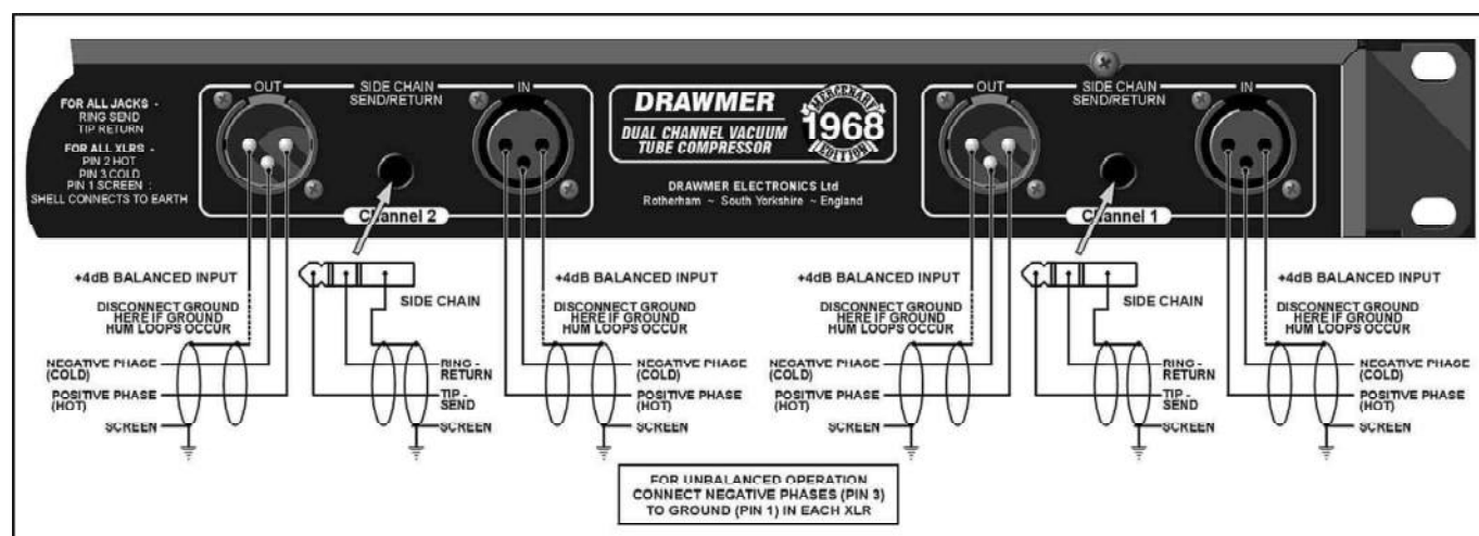
fig. 1 1968 WIRING
