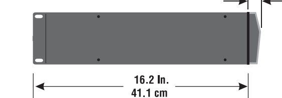
Abb. 2.1 Abmessungen
