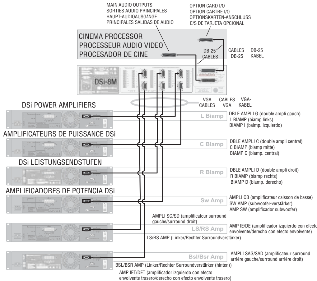
Figure 2.3 Connexion des amplificateurs DSi au panneau de surveillance DSi-8M en utilisant les connecteurs HD-15
