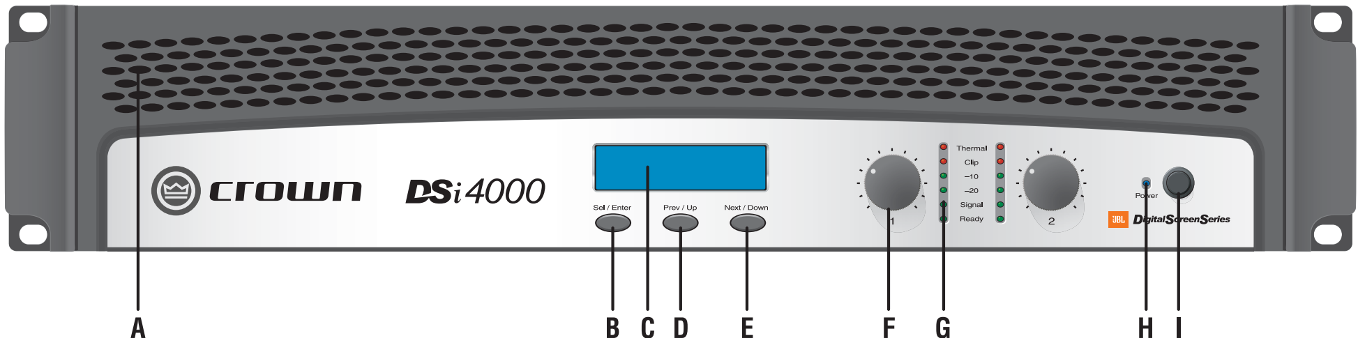
Abb. 3.1 Vorderseitige Regler und Anzeigen
