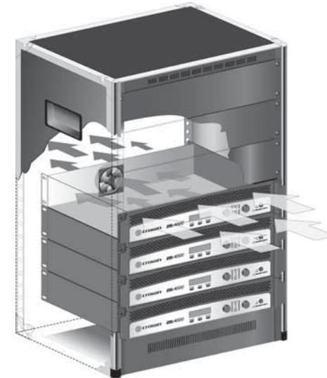
Figura 2.2 Flujo de Aire
