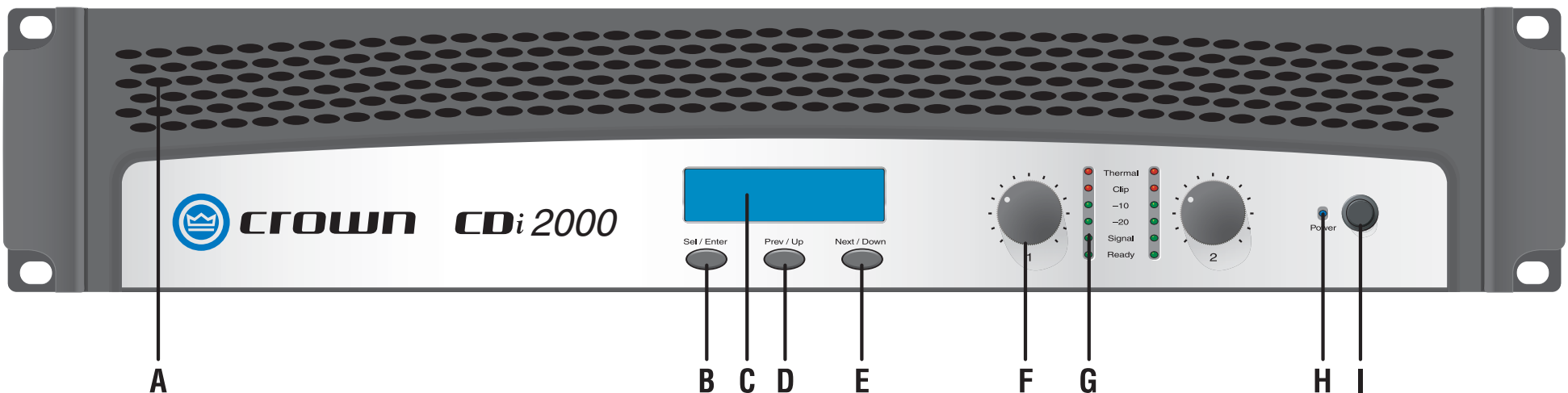
Abb. 3.2 Vorderseitige Regler und Anzeigen
