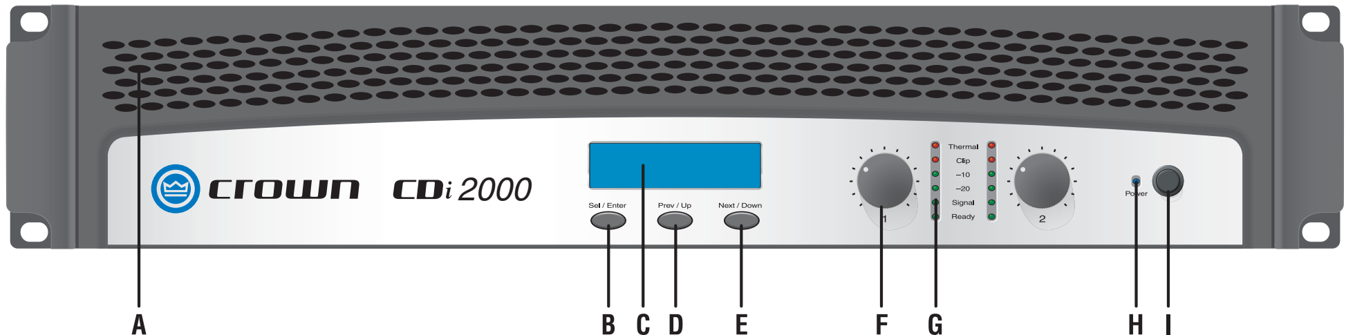
Figure 3.1 Commandes et indicateurs de façade
