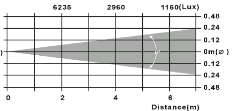
RLR-835 : Lampe 150W ; Ouverture 9°
