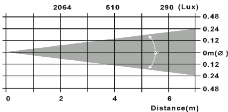
SCN-835 : Lampe 150W ; Ouverture 9°
