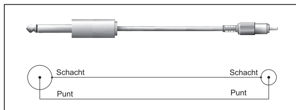
Afb. 4.4: Adapterkabel mono
