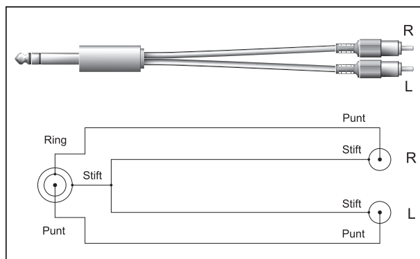
Afb. 4.3: Adapterkabel stereo
