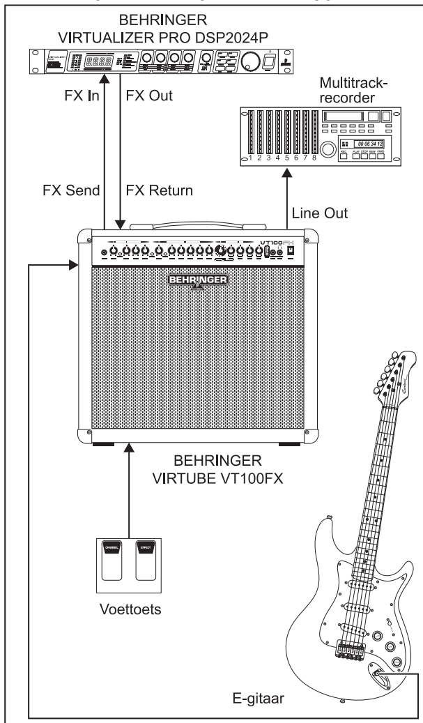
Afb. 3.2: Opnameset-up met de VT100FX
