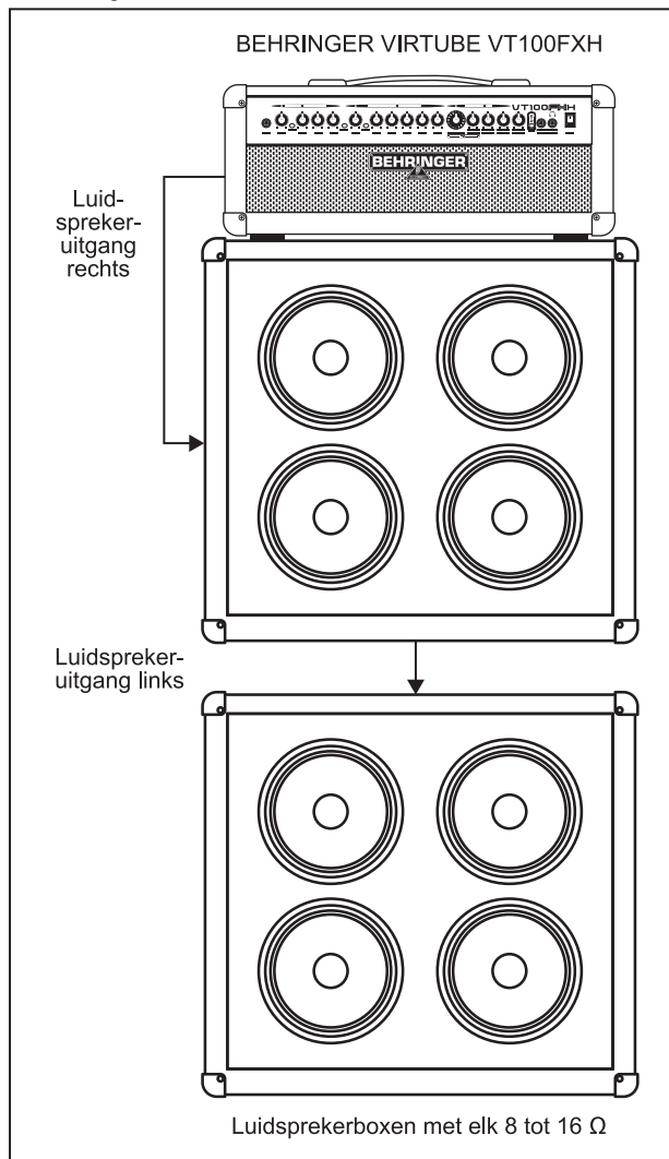
Afb. 3.4: VT100FXH met twee luidsprekerboxen
