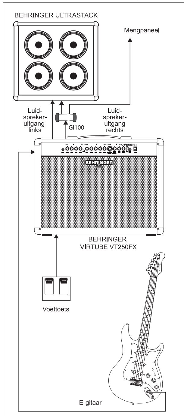
Afb. 3.3: Set-up met de VT250FX in combinatie met een luidsprekerbox
