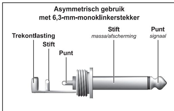
Afb. 4.1: 6,3 mm monostekker
