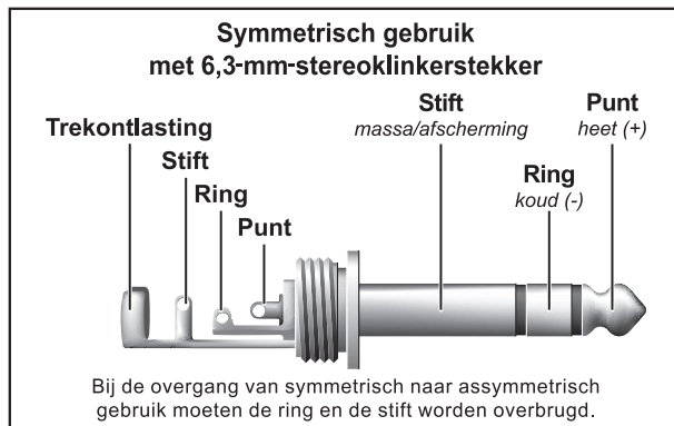
Afb. 4.2: 6,3 mm stereostekker
