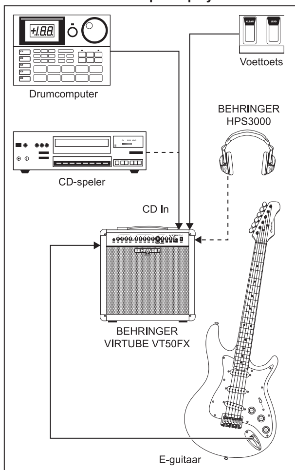
Afb. 3.1: Standaardset-up met de VT50FX
