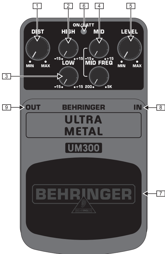
Aanzicht bovenkant
