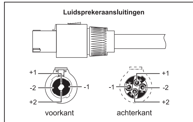
Fig. 4.1: Luidsprekeraansluitingen
