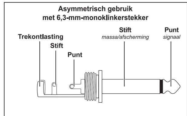
Fig. 4.4: 6,3-mm-monoklinkerstekker
