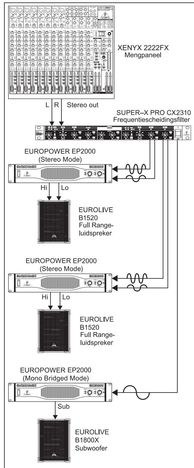
Fig. 3.7: Stereo Bi-amp-bedrijf met aparte subwoofer
