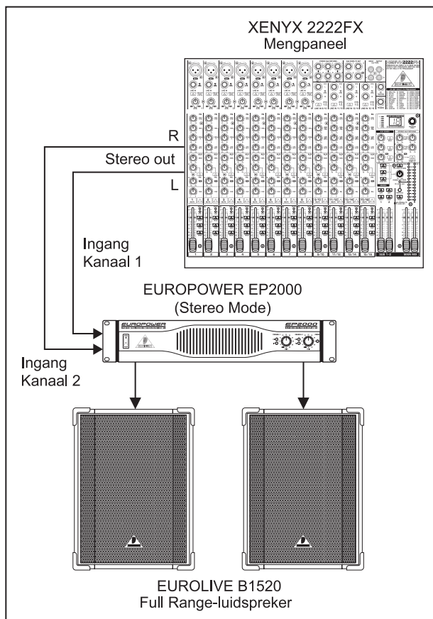
Fig. 3.1: Tweekanaalsbedrijf
