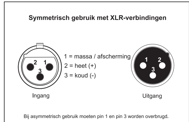
Fig. 4.3: XLR-verbindingen
