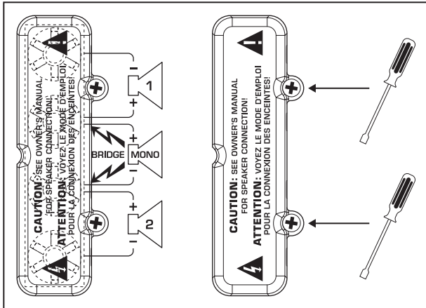
Fig. 4.2: Kunststofafdekking over de aansluitklemmen
