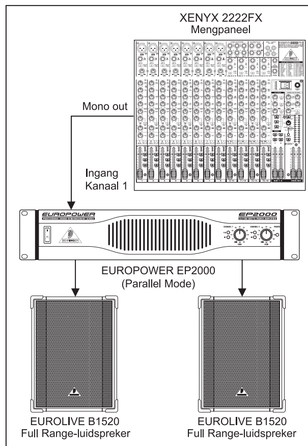
Fig. 3.3: Parallele modus
