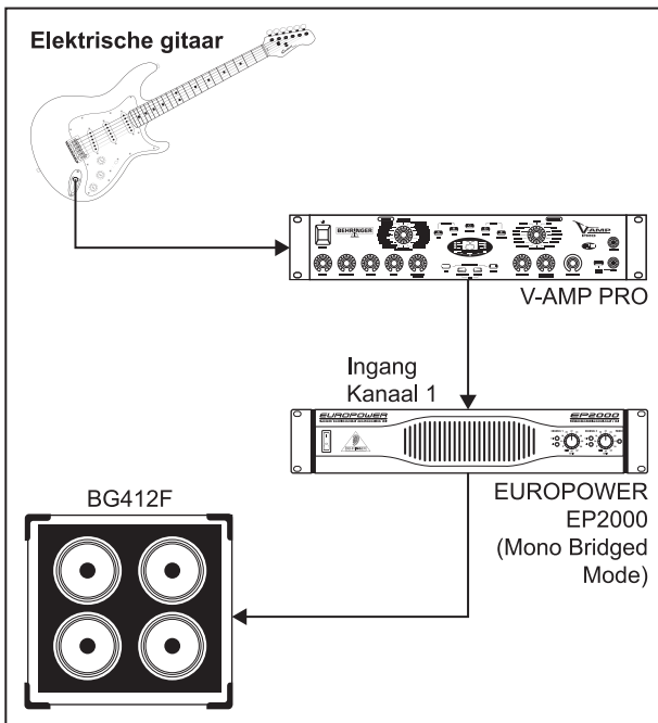
Fig. 3.5: Gebruik als monobrug
