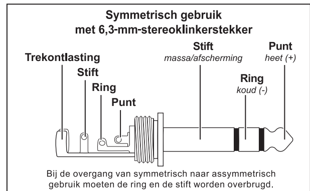
Fig. 4.5: 6,3-mm-stereoklinkerstekker
