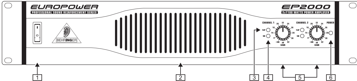
Fig. 2.1: De bedieningselementen aan de voorkant
