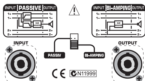
Afb. 1.1: Aansluitingen voor de subwoofer (E1800X)
