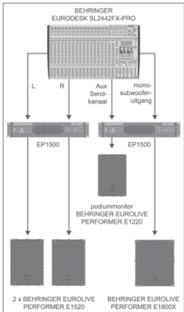
Afb. 6.1: Stereoweergave met podiummonitor en subwoofe
