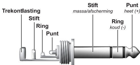
Afb. 4.3: 6,3-mm-stereoklinkerstekker
