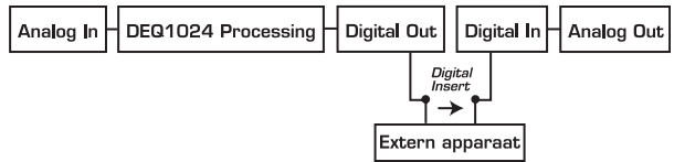
Afb. 2.6: Signaalstroom in de POST EQ-modus
