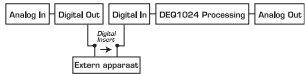
Afb. 2.5: Signaalstroom in de PRE EQ-modus
