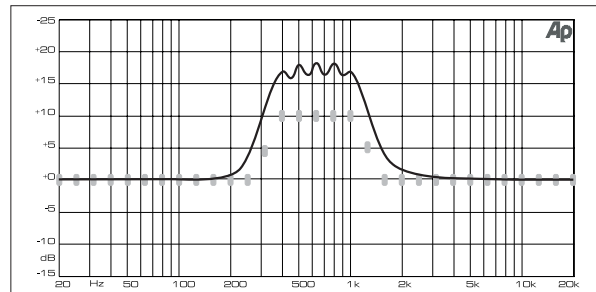
Afb. 2.2: Grafische equalizer zonder correctie van het frequentiekaracteristiek
