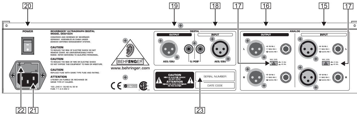
Afb. 2.7: De bedieningselementen en aansluitingen aan de achterkant
