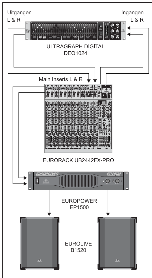
Afb. 3.1: De ULTRAGRAPH DIGITAL DEQ1024 als som-equalizer
