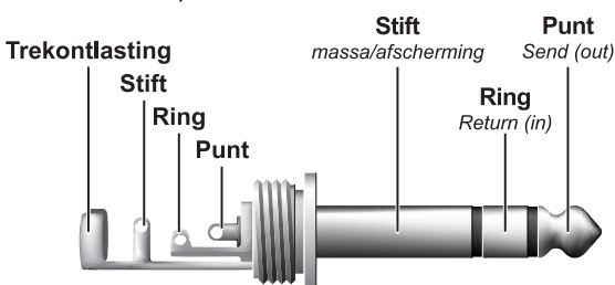
Afb. 4.4: 6,3-mm-stereoklinkerstekker voor insert-kabels
