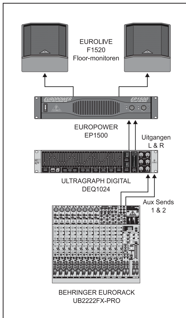
Afb. 3.2: De ULTRAGRAPH DIGITAL DEQ1024 in een monitorinstallatie
