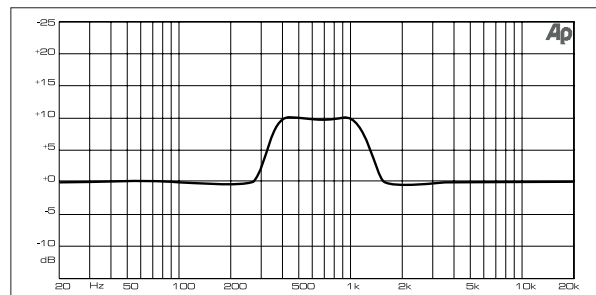
Afb. 2.3: Grafische equalizer met correctie van het frequentiekaracteristiek (TRUE CURVE)
