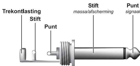
Afb. 4.2: 6,3-mm-monoklinkerstekker
