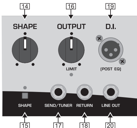
Afb. 2.3: Bedieningselementen aan de voorkant (sectie 3)
