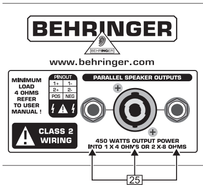
Afb. 2.5: De achterkant van de BX4500H (sectie 2)
