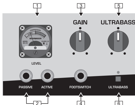
Afb. 2.1: Bedieningselementen aan de voorkant (sectie 1)
