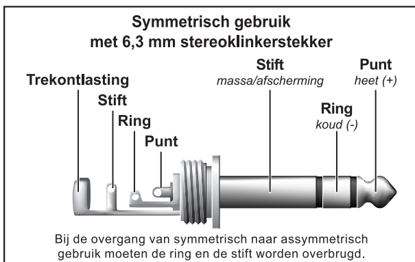
Afb. 7.2: 6,3-mm-stereoklinkerstekker
