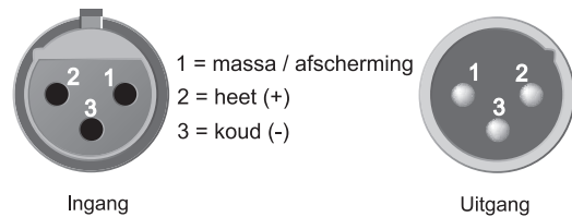
Afb. 7.3: XLR-verbindingen
