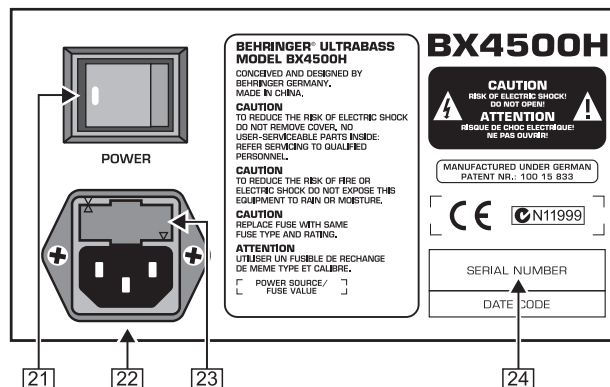
Afb. 2.4: De achterkant van de BX4500H (sectie 1)
