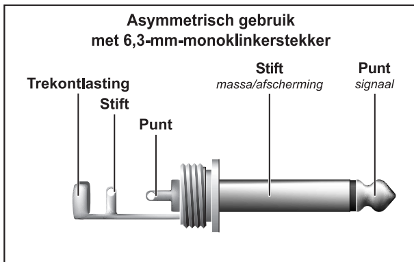
Afb. 7.1: 6,3-mm-monoklinkerstekker
