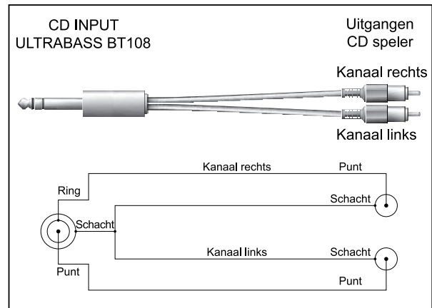
Afb. 4.3: Adapterkabel stereo
