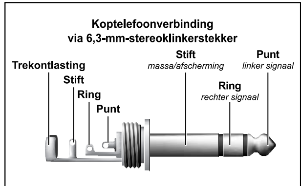
Afb. 4.2: Bedrading van de stereoklinkerstekker voor de koptelefoon en de cd INPUT
