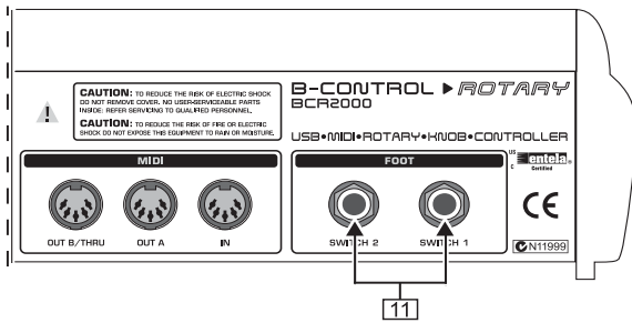
Afb. 3.3: De voetschakelaaraansluitingen van de BCR2000
