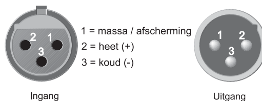
Afb. 4.1: XLR-aansluitingen
