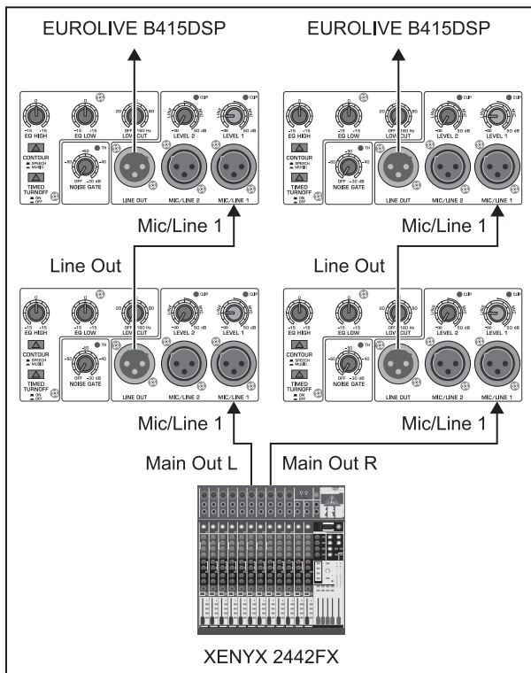
Afb. 3.3: Aaneenschakeling van meerdere B415DSP's
