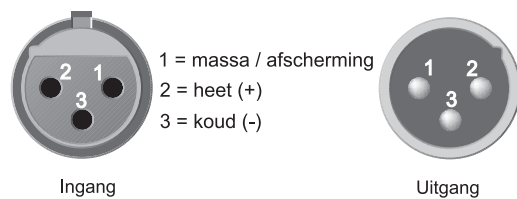
Afb. 4.1: XLR-aansluitingen
