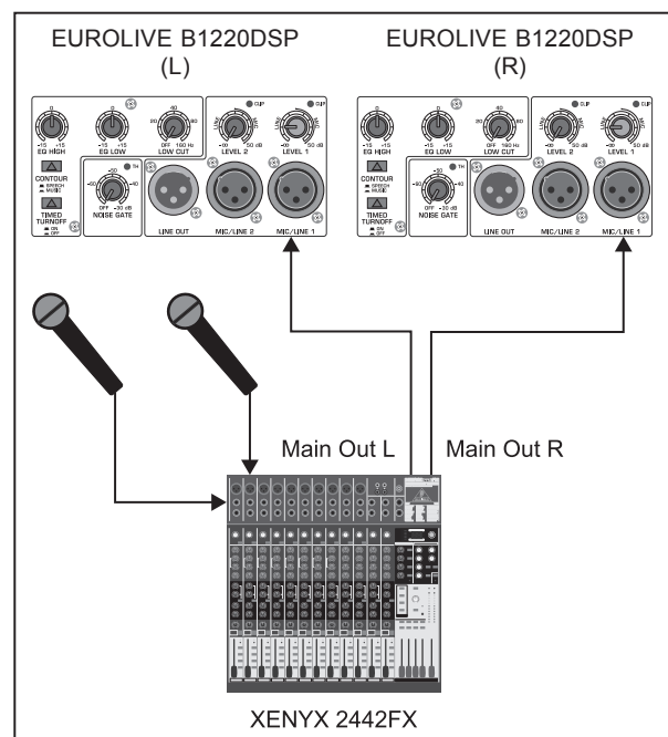
Afb. 3.2: Aansluiting van een mengpaneel
