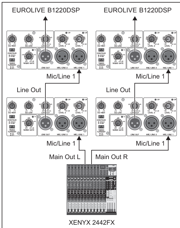
Afb. 3.3: Aaneenschakeling van meerdere B1220DSP's
