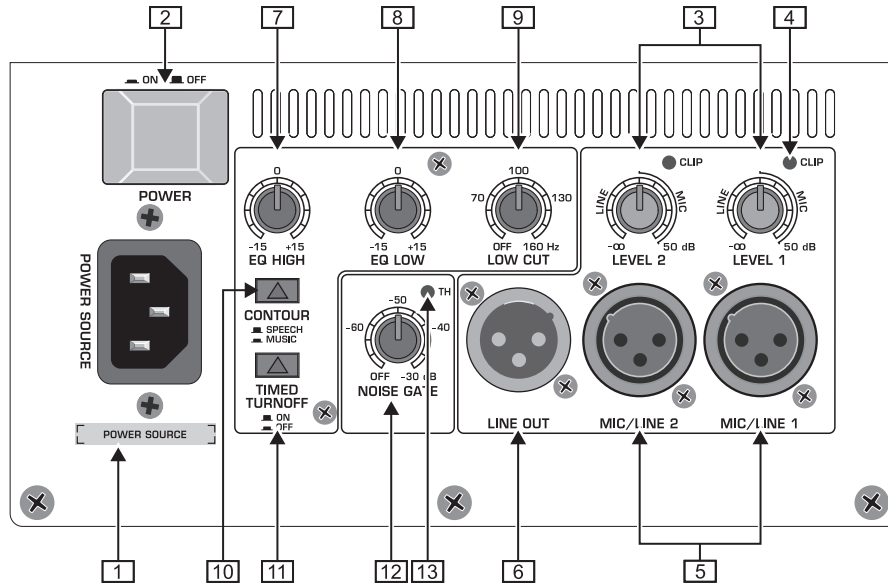
Afb. 2.1: Bedieningselementen en aansluitingen op de achterzijde
